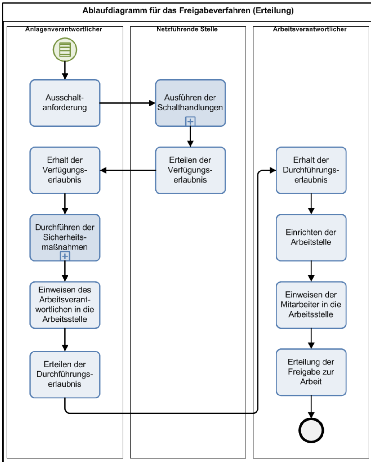
Ablaufdiagramm für die Rücknahme einer Freigabe (Hoch- und Mittelspannung)
